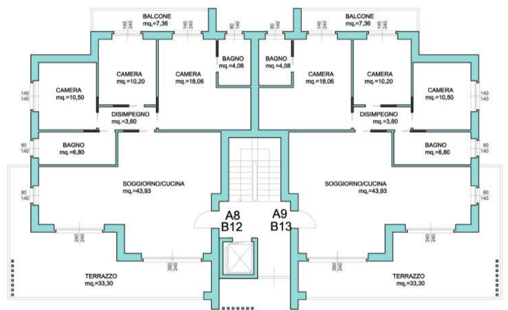
PIANO PRIMO 1:200
