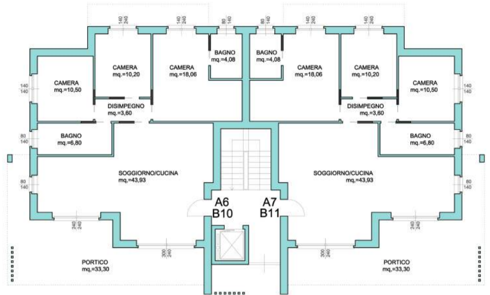
PIANO TERRA 1:200
