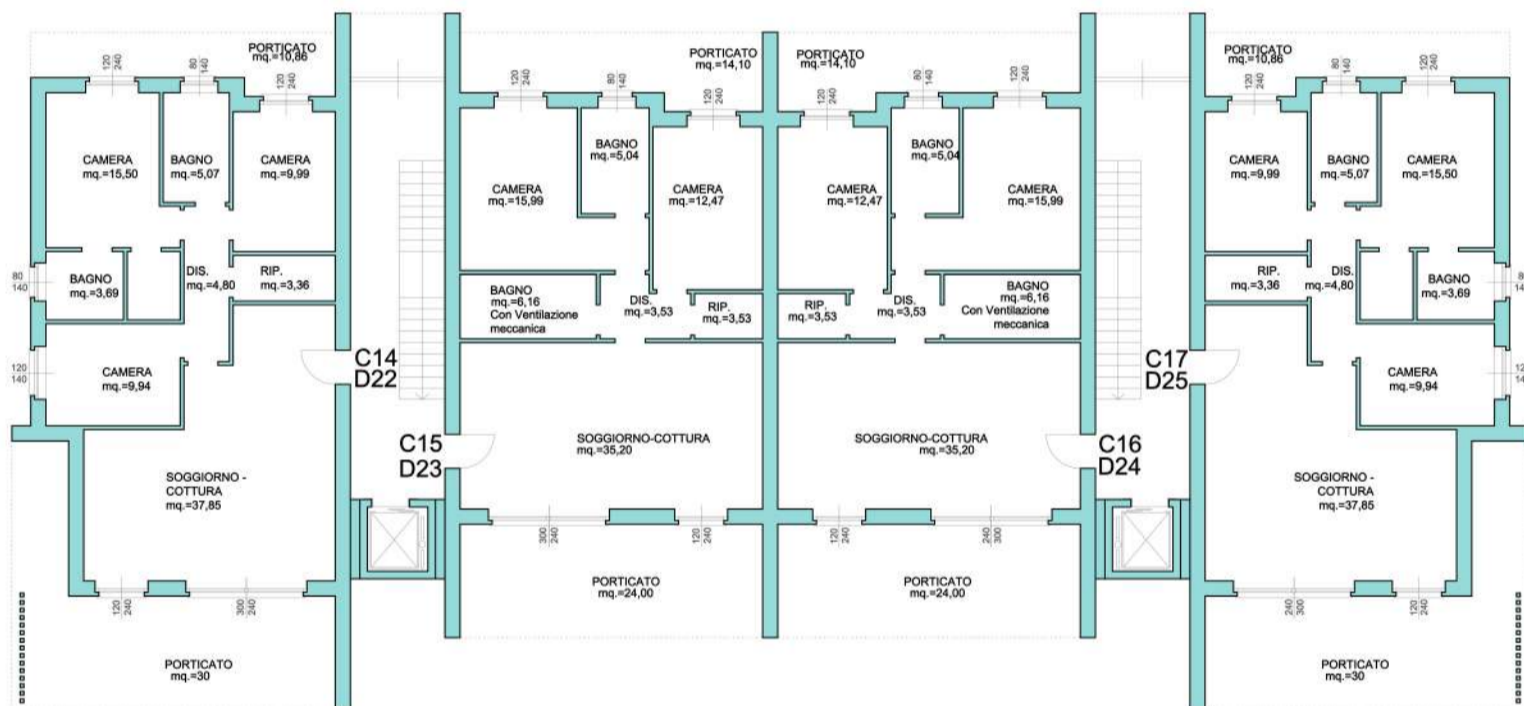
PIANO TERRA 1:200
