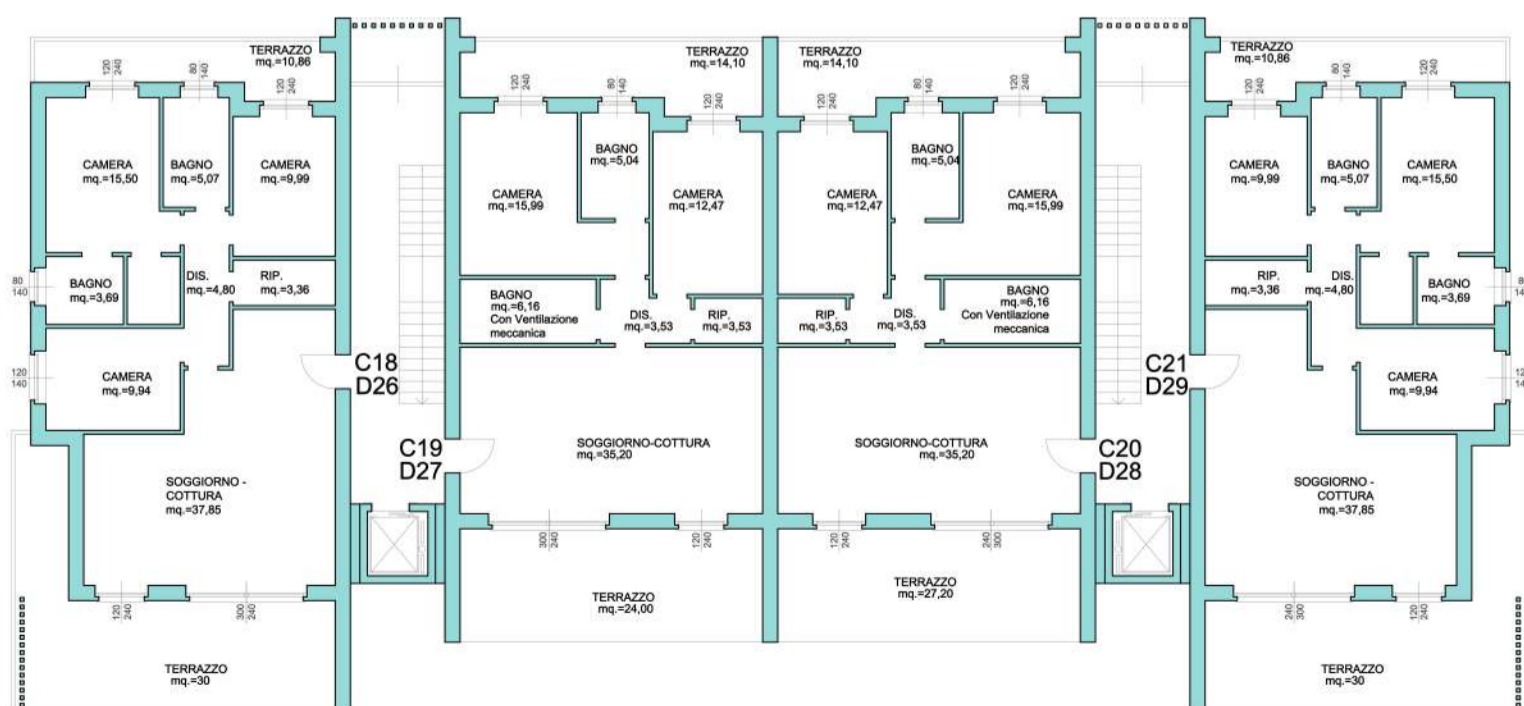
PIANO PRIMO 1:200
