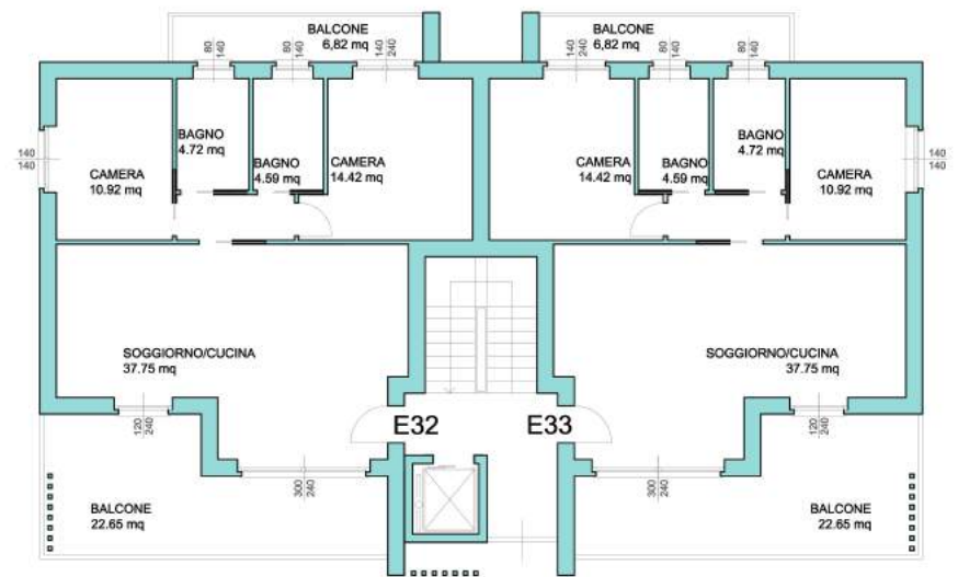
PIANO PRIMO 1:200
